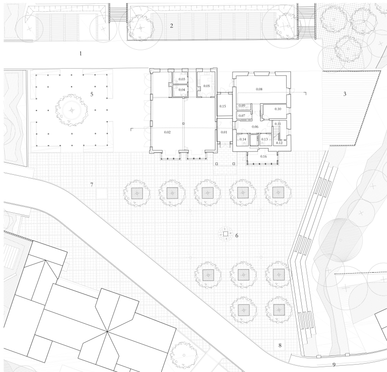
Rzut partetu Nowego Młyna i zagospodarowanie Placu Przedmłyńskiego
