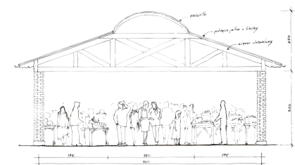
Przekrój typowy targowiska, 1:75
