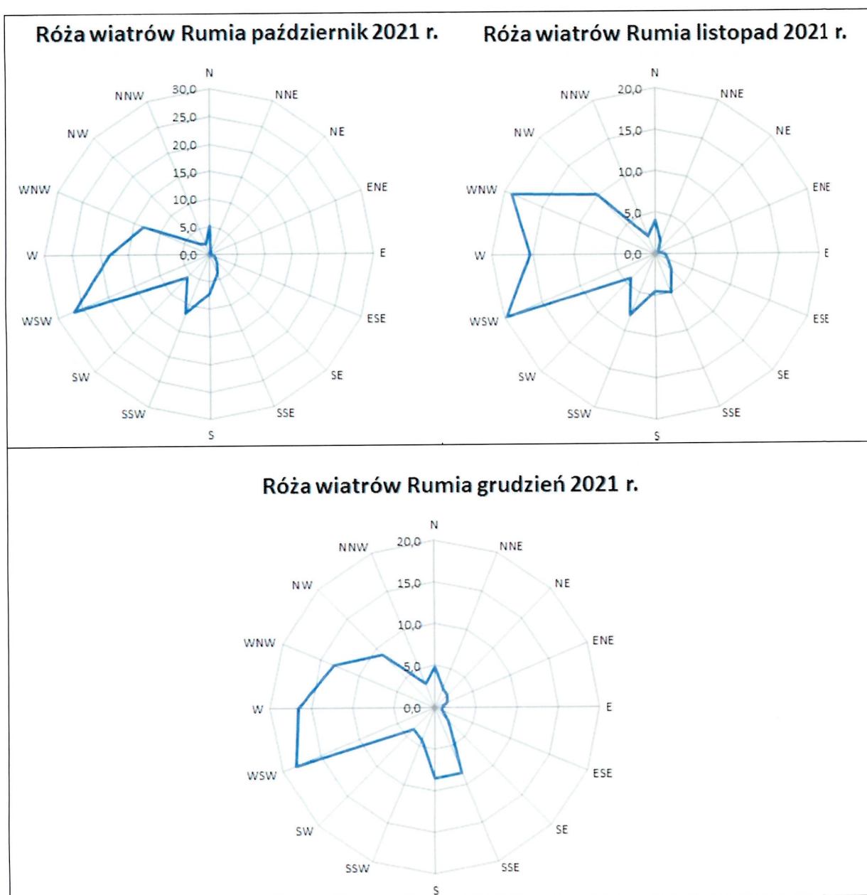
Rys.2 Róże wiatrów w miesiącach październik – grudzień 2021 rok.
