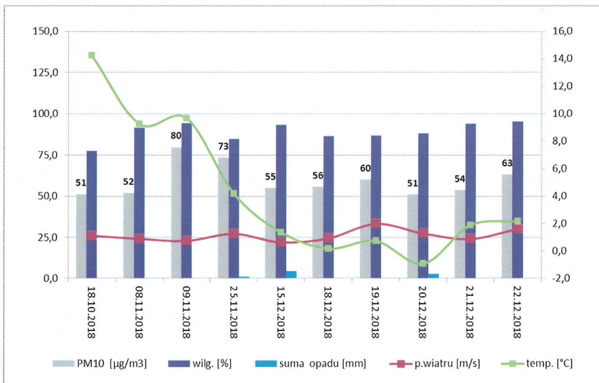
Rys.10 Przekroczenia wartości pyłu zawieszonego PM_{10} na tle średnich warunków meteorologicznych w Rumi w okresie od 04.07.2018 r. do 31.12.2018 r.
