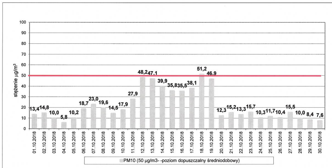
Ryc.6 Średniodobowe wartości stężeń pyłu PM 10
