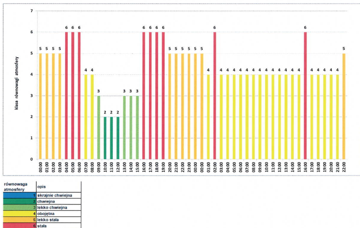
Rys.9 Klasy równowagi atmosfery w dniu wystąpienia epizodu (8-9.11.2018) z maksymalną wartością średniodobową tj. 9 listopada 2018 roku.
