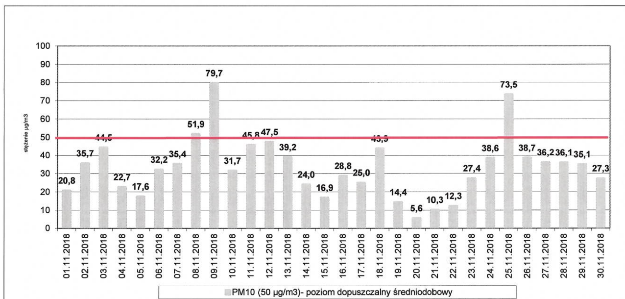
Ryc.7 Średniodobowe wartości stężeń pyłu PM 10 .
